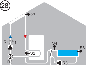
Solare piscina, accumulatore, scambiatore
