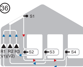
Solare con 3 accumuli e 3 pompe
