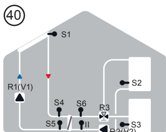
Solare con scambiatore e 2 accumuli
