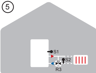
Incremento ritorno
