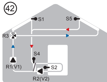
Solare est-ovest, scambiatore e 2 pompe
