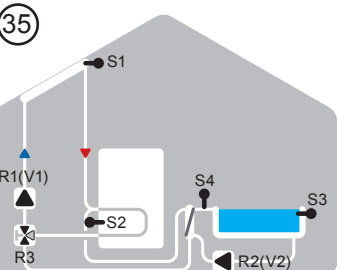
Solare con piscina, accumulatore, scambiatore
