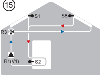
Solare + 2 collettori
