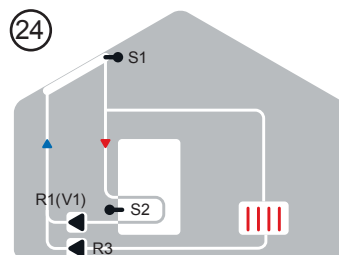
Solare + raffreddamento 2
