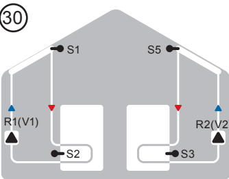
Doppio solare
