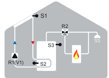
Solare + termostato come valvola
